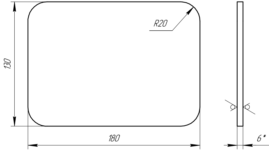
Дет. поз. 2
